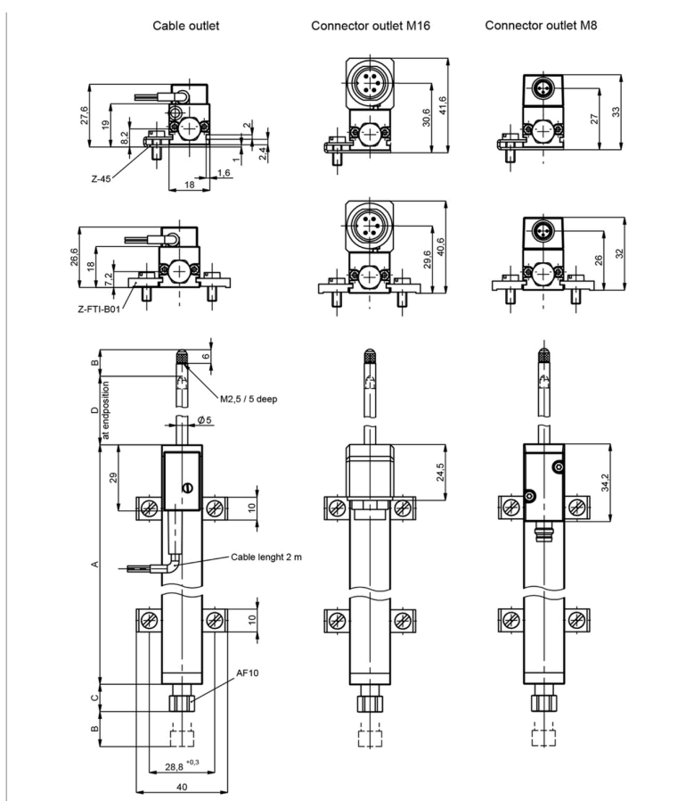
Plano dimensional: salida de cable, conector M16 y conector M8. Medidas en mm.
