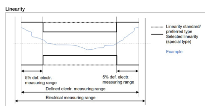
Linealidad
