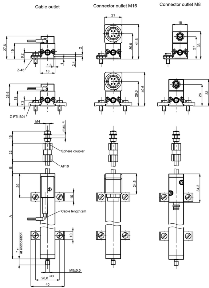
Plano dimensional: salida de cable, conector M16 y conector M8. Medidas en mm.
