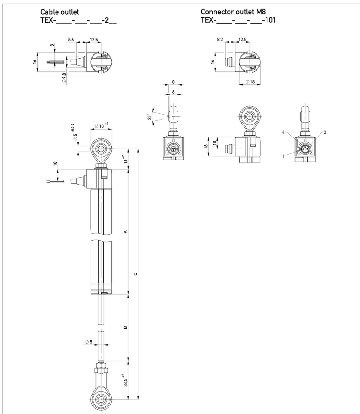
Plano dimensional: salida de cable y salida de conector M8. Medidas en mm.
