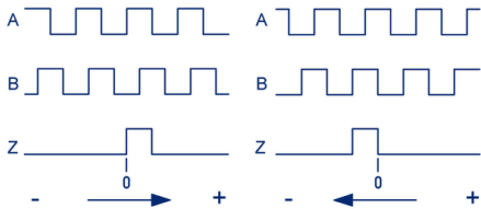
Señales A, B y Z
