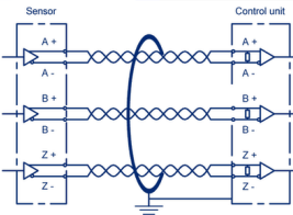
Conexión RS422 (A/B/Z)
