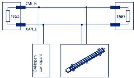
Bus CANopen con terminación de 120 Ω
