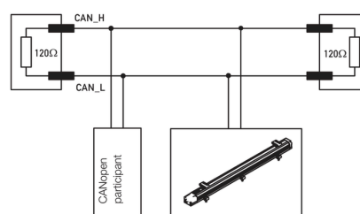
Bus CANopen con terminación de 120 Ω
