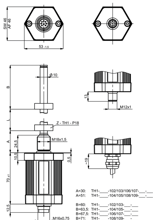
Plano dimensional. Medidas en mm.
