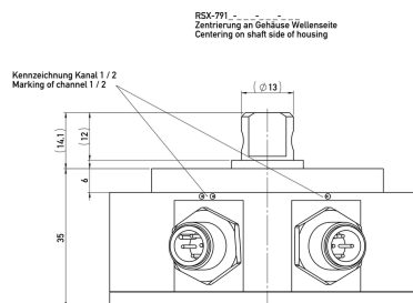
RSX-791: centrado en el lado del eje. Medidas en mm.
