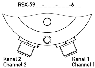
Conector, dos canales (-6). Medidas en mm.
