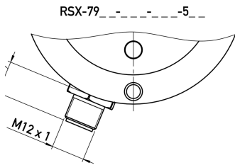
Conector, un canal (-5). Medidas en mm.
