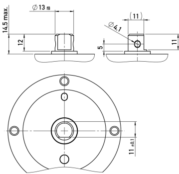
Eje 1: Ø 13 x 12 mm. Medidas en mm.
