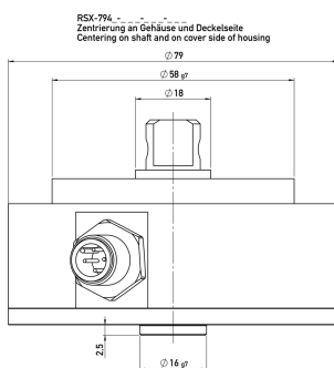
RSX-794: centrado en el eje y en la tapa. Medidas en mm.
