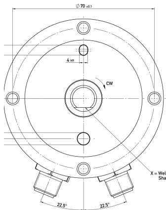
Vista inferior. Medidas en mm.
