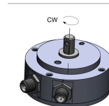
Marca del eje respecto al orificio de indexado
