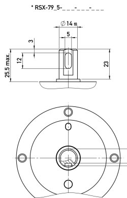
Eje 5 (bajo pedido). Medidas en mm.
