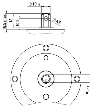
Eje 3: Ø 10 x 16 mm. Medidas en mm.
