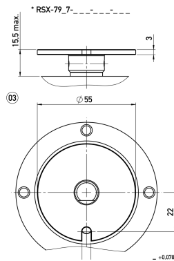
Eje 7 (bajo pedido). Medidas en mm.
