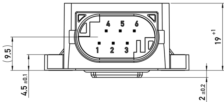
Vista del conector
