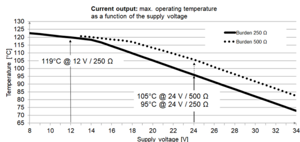
Temperatura máx. en función de Ub y de la carga (corriente)
