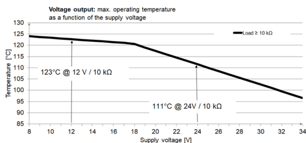
Temperatura máx. en función de Ub (tensión)
