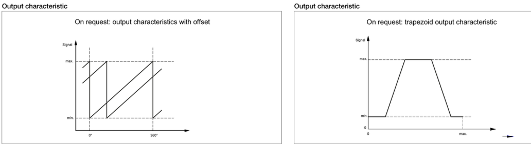
Características de salida bajo pedido
