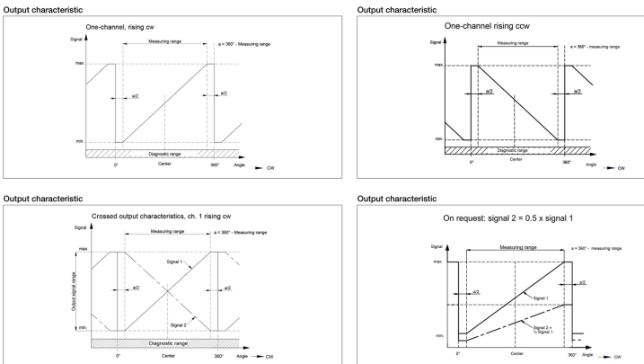
Características de salida
