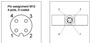
Conector M12, 4 polos, codificación A
