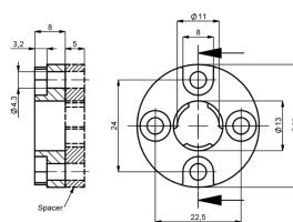
Fijación M4 (Ø 32 mm, con o sin distanciador) Z-TH1-P19 (Art. 400005698) · Z-TH1-PD19 (Art. 400107117)
