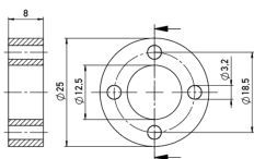
Fijación tornillos M3 (Ø 25 mm, peso ca. 12 g) Z-TH1-P18 (Art. 400005697)
