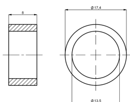
Fijación por arandela de presión y anillo elástico (Ø 17,4 mm) Z-TH1-P30 (Art. 400106139)
