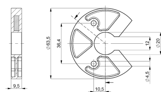
Forma en U tornillos M4 (Ø 63,5 mm) Z-TH1-P25 (Art. 400105076)
