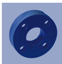
Fijación M4 (Ø 32 mm, con o sin distanciador) Z-TH1-P19 (Art. 400005698) · Z-TH1-PD19 (Art. 400107117)
