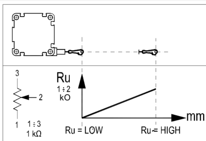
Esquemas de electrónica de salida
