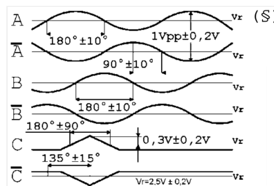
Sinusoidal 1 Vpp
