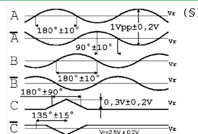
Sinusoidal 1 Vpp
