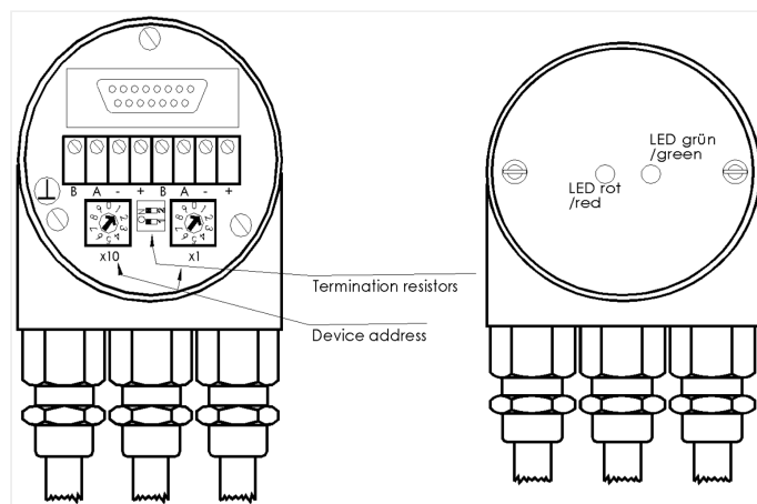
Detalle de Conexión e Interfaz Profibus-DP (Tapa 3PG con 2 LED)
