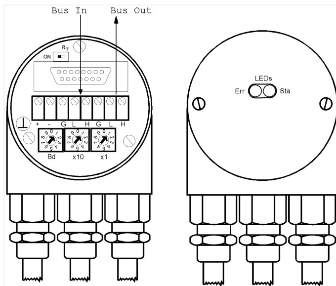
Tapa de conexión 3PG con 2 LED
