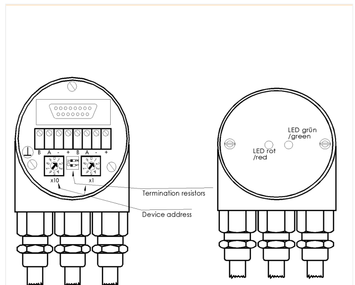
Tapa de conexión 3PG con 2 LED
