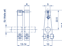
Horquilla sin holgura Z-105-G-6
