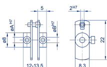
Horquilla con poca holgura Z-103-G-3
