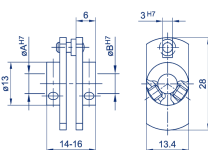
Horquilla con poca holgura Z-104-G-6
