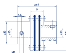
Acoplamiento sin holgura Z-110-G-10
