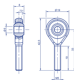
Rótula para vástago TP1 Z-G02
