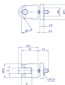
Cabezal de rodillo Z-R50
