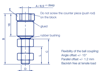
Acoplamiento articulado Z-301-M6/M6, M6/M4, M5/M5
