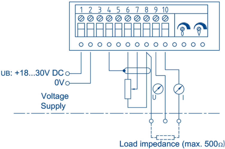
Esquema de conexiones del fabricante.
