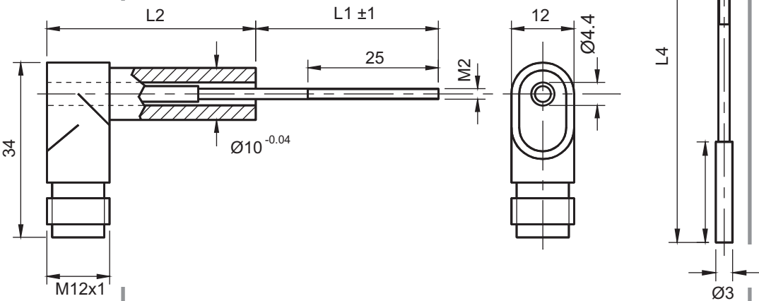
Dimensiones palpador:
