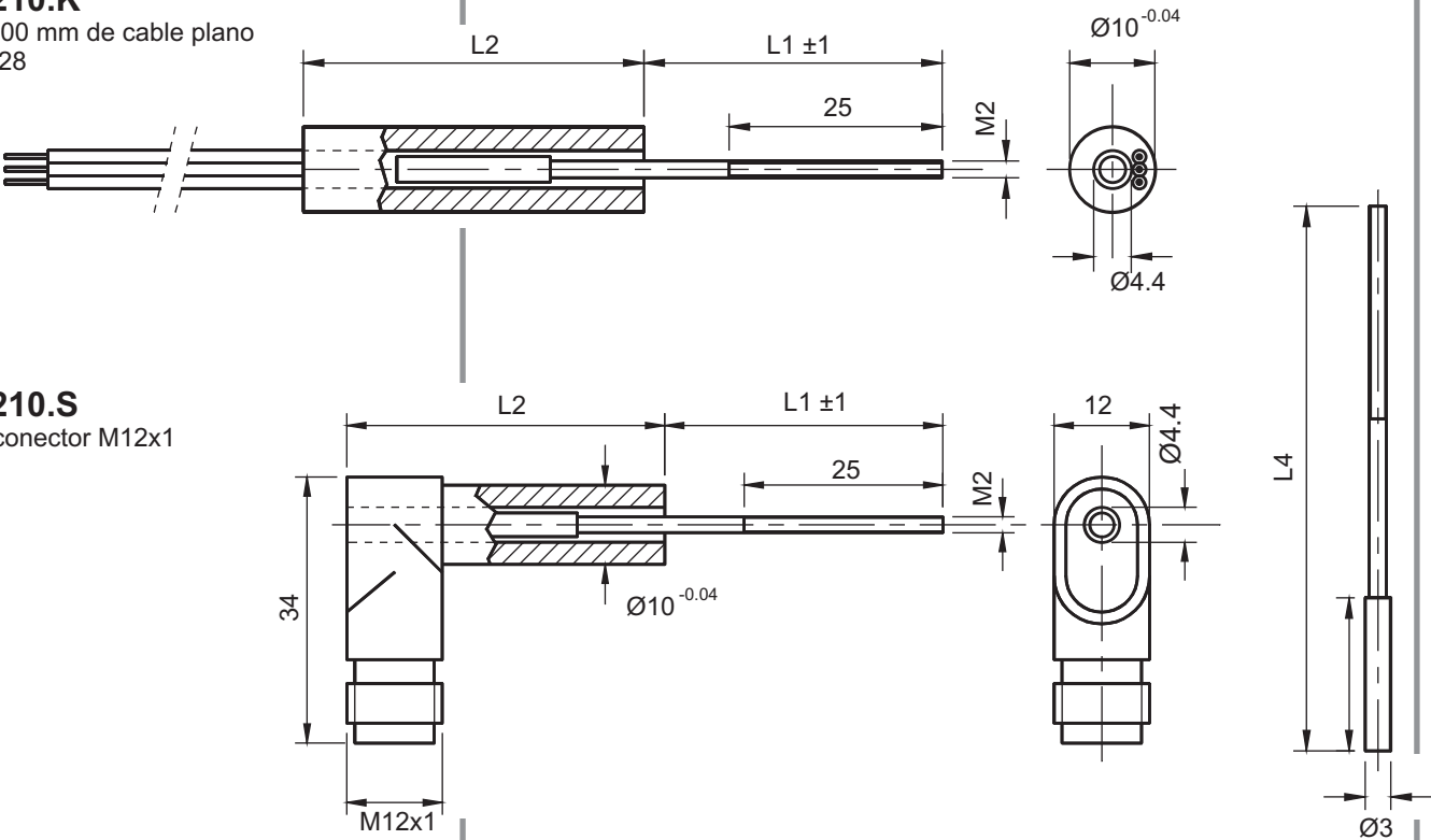
Dimensiones palpador:
